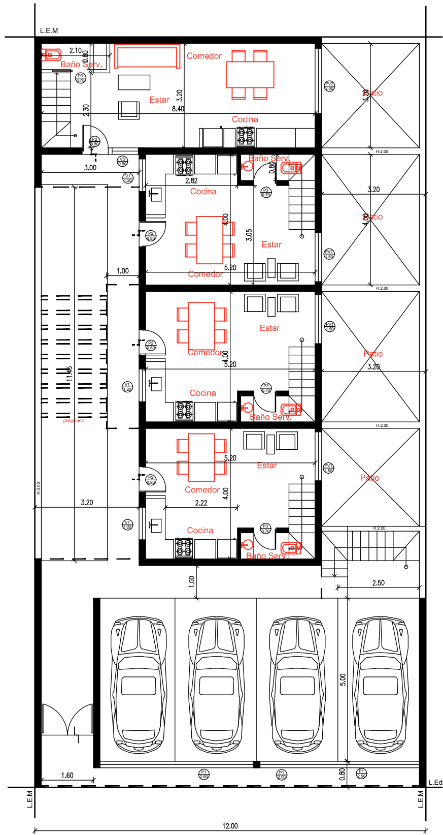
L.C.V. Planta baja general esc 1:100
